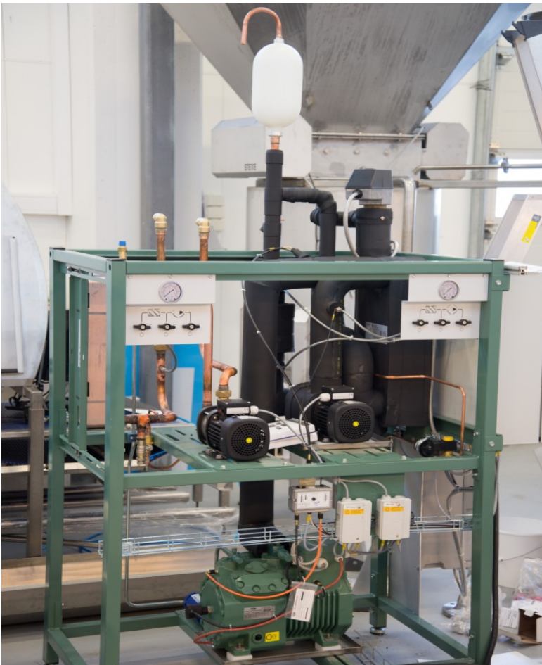
Figur 4: Kjøleanlegget
