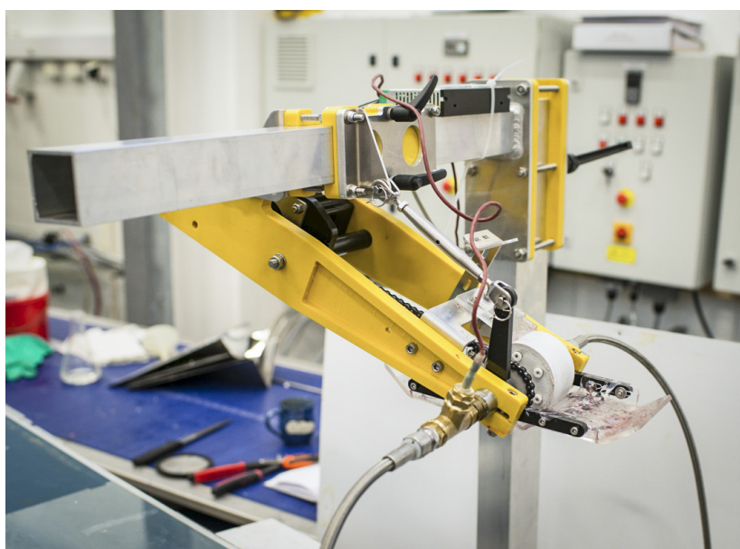
Figur 3: modifisert prototype
